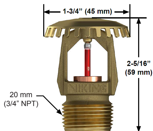
Rysunek nr 2: Wymiary tryskacza VK531
