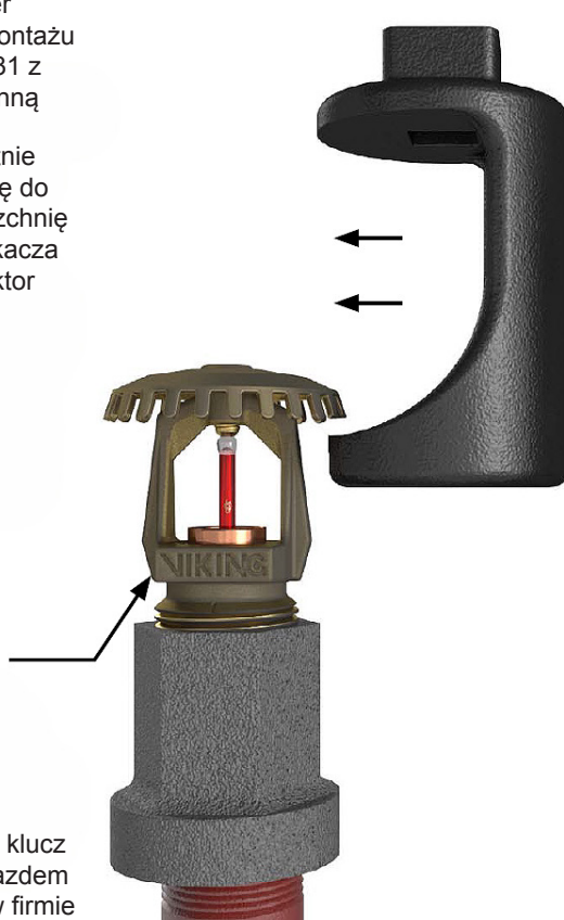
Rysunek nr 3: Klucz nr 11663W/B dla tryskacza VK531 z powłoką ochronną.
