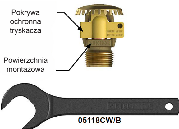
Rysunek nr 1: Tryskacz VK531 i klucz nr 05118CW/B
