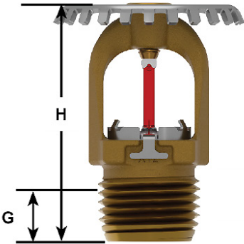
Rysunek 2 - Wymiary
