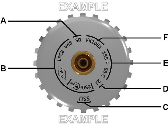
Rysunek 1 - Oznakowania
