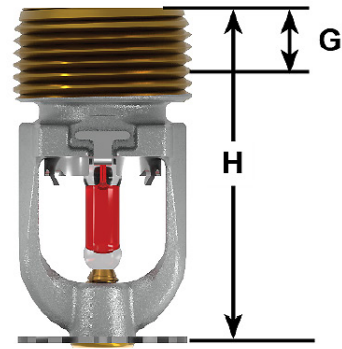
Rysunek 2 - Wymiary
