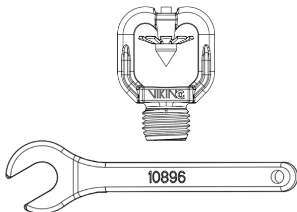
Rys. 4 Standardowy klucz nr 10896W/B
