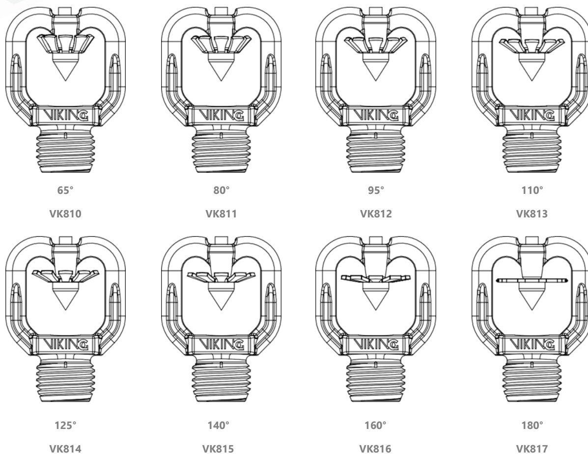
Rys. 3 Kąty wypływu
