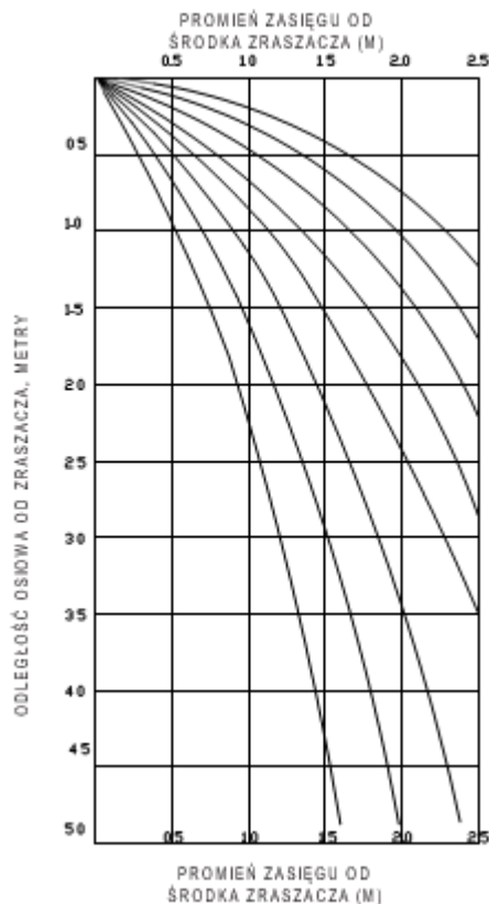
Wykres 1b. Charakterystyka wypływu (metry)
