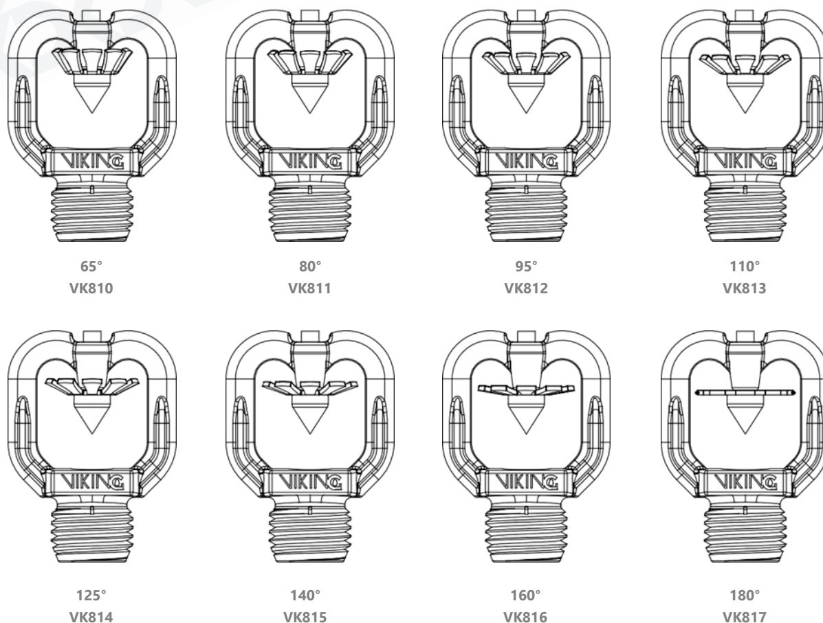
Rys. 3 Kąt wypływu
