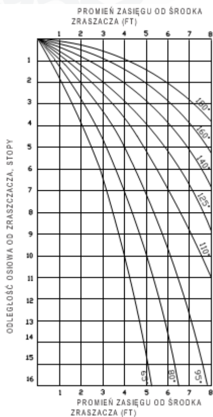
Wykres 1a. Charakterystyka wypływu (stopy)
