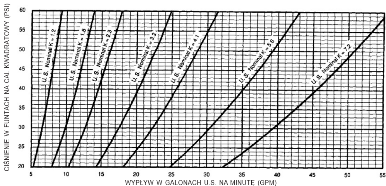
Wykres 2. Nominalne charakterystyki wypływu
