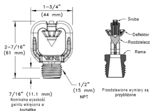
Rys. 5 Wymiary zraszacza
